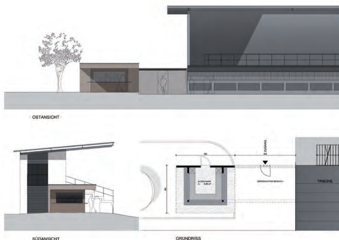
Die Planansichten der neuen Überdachung samt Ausschank.
