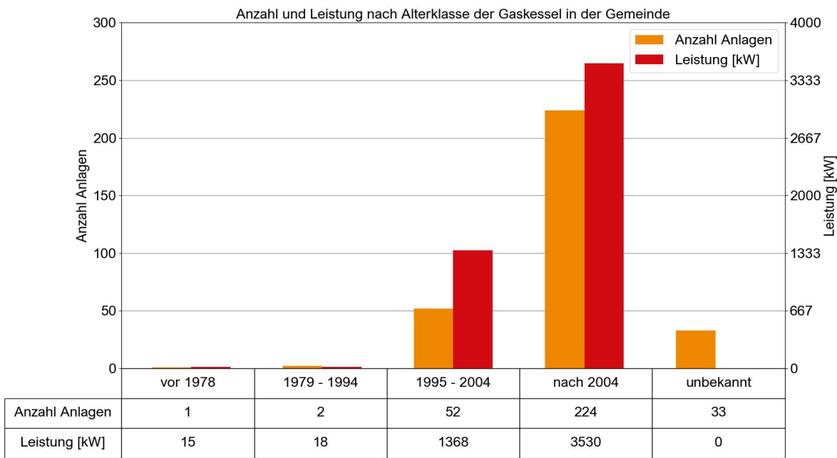
Abbildung 7: Anzahl und Leistung nach Altersklasse der Gaskessel
