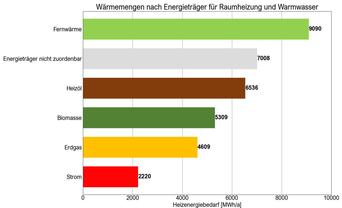
Abbildung 4: Wärmemengen nach Energieträger für Raumheizung und Warmwasser
