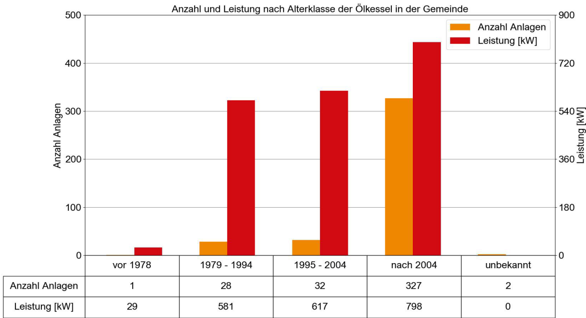
Abbildung 6: Anzahl und Leistung nach Altersklasse der Ölkessel
