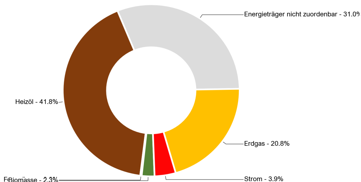
Abbildung 5: Anteil der Treibhausgasemissionen nach Energieträger
