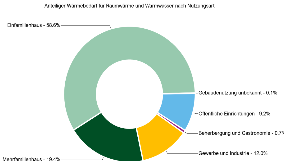
Abbildung 3: Anteiliger Wärmebedarf für Raumwärme und Warmwasser nach Nutzungsart
