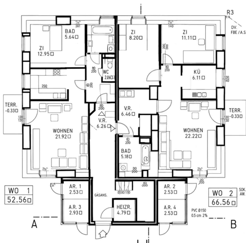
Grundriss Erdgeschoss
