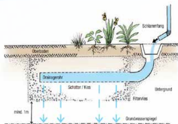
Abb. 26: Schematischer Aufbau einer Rohr-Rigolenversickerung © Magistrat der Stadt Wien, Wiener Umweltschutzabteilung
