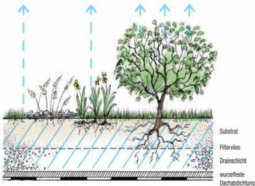
Abb. 10: Intensive Dachbegrünung © Magistrat der Stadt Wien, Wiener Umweltschutzabteilung
