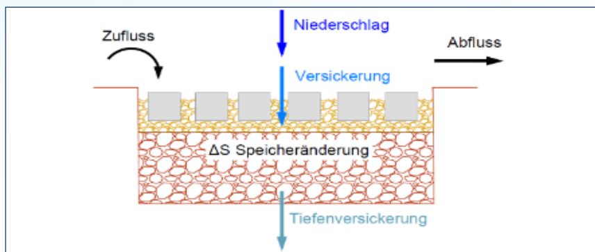
Abb. 15: Versickerung bei wasserdurchlässigen Belägen © Bundesministerium Nachhaltigkeit und Tourismus
