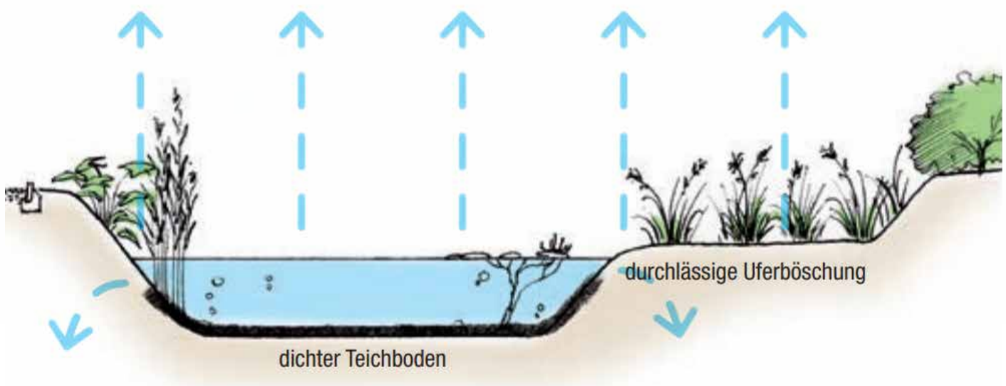
Abb. 39: Aufbau eines Versickerungsteiches © Magistrat der Stadt Wien, Wiener Umweltschutzabteilung
