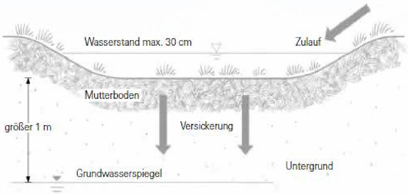
Abb. 21: Schematischer Aufbau einer Muldenversickerung © Bayerisches Landesamt für Umwelt
