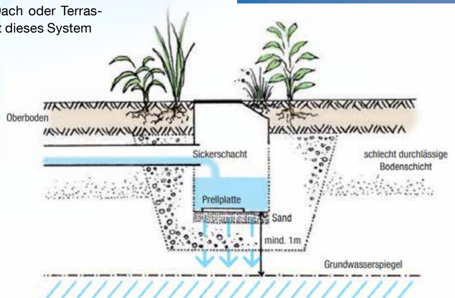
Abb. 35-37: Bau eines Sickerschachtes © Adobe.Stock.com
