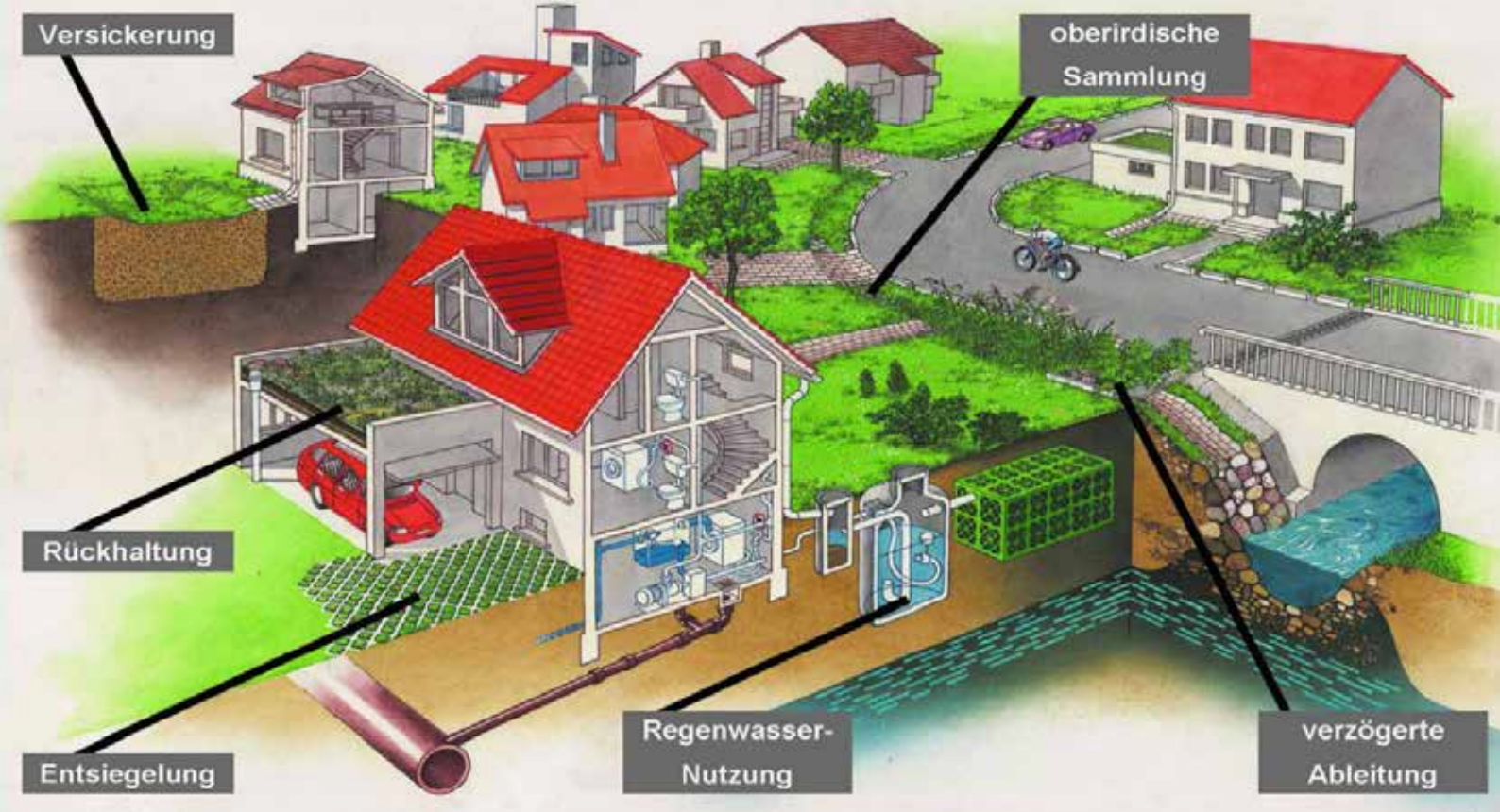
Abb. 1: Wesentliche Elemente der naturnahen Regenwasserbewirtschaftung © Bayerisches Landesamt für Umwelt
