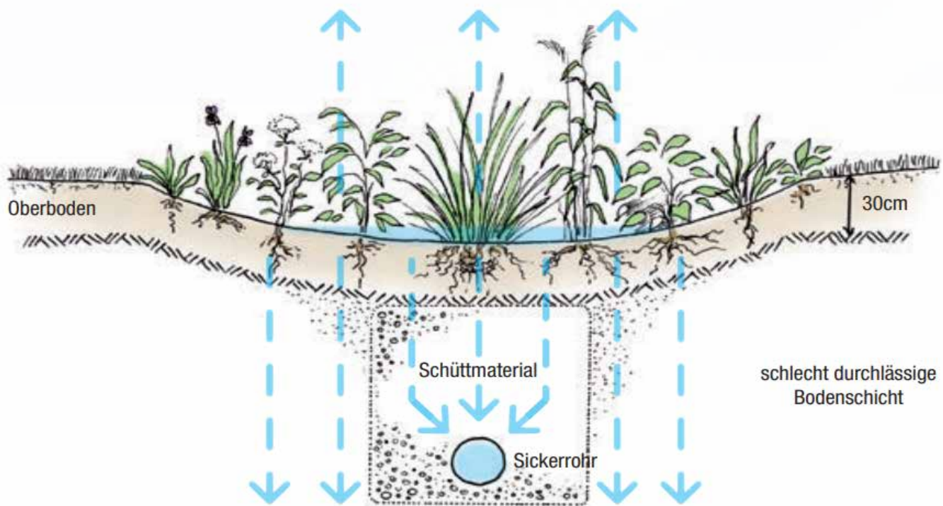
Abb. 31: Mulden-Rigolenversickerung © Magistrat der Stadt Wien, Wiener Umweltschutzabteilung
