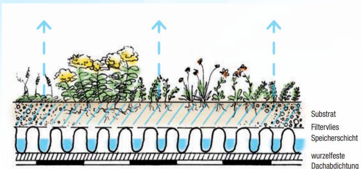
Abb. 8: Extensive Dachbegrünung mit Retentionsdach © Magistrat der Stadt Wien, Wiener Umweltschutzabteilung
