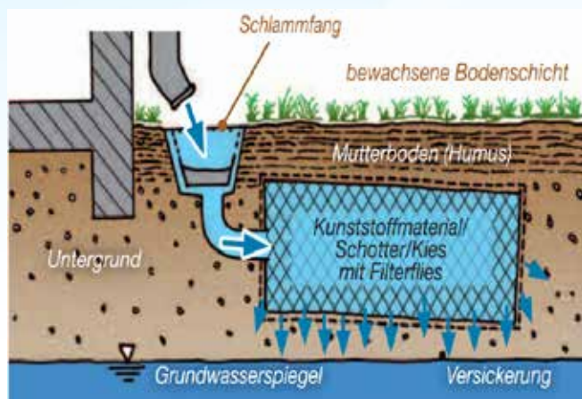
Abb. 25: Rigol-Versickerung © Amt der NÖ Landesregierung, Abteilung Siedlungswasserwirtschaft
